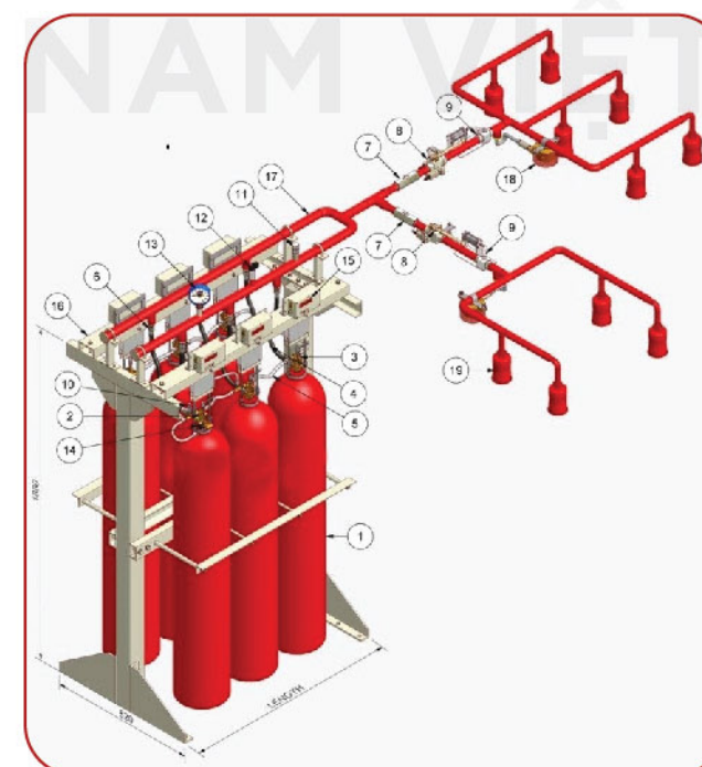
HỆ THỐNG CHỮA CHÁY TỰ ĐỘNG FM-200 (HFC-227EA)
